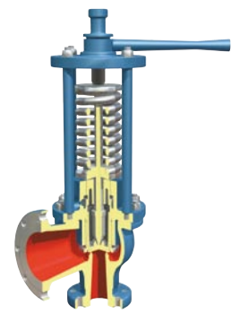
A7000 系列 (锅炉用) ISO 4126 (+3% 过压) 短喷嘴 尺寸 : 2" - 6" 整定压力: 最大 150 barg 温度 : 最高 +565°C 材质 : 碳钢 - 合金钢 - 不锈钢
